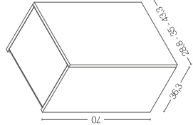
PENSILE A GIORNO JOLLY JOLLY OPEN WALL UNIT
