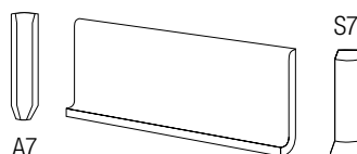
*zoccolo a raccordo a becco civetta cove base with rounded edge plinthe à gorge bord arrondi hohlkehlsocbel mit abgerundeter Kante
