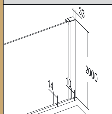
TOGA TW-1
