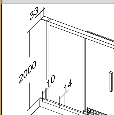
TOGA TN/TI/TC
