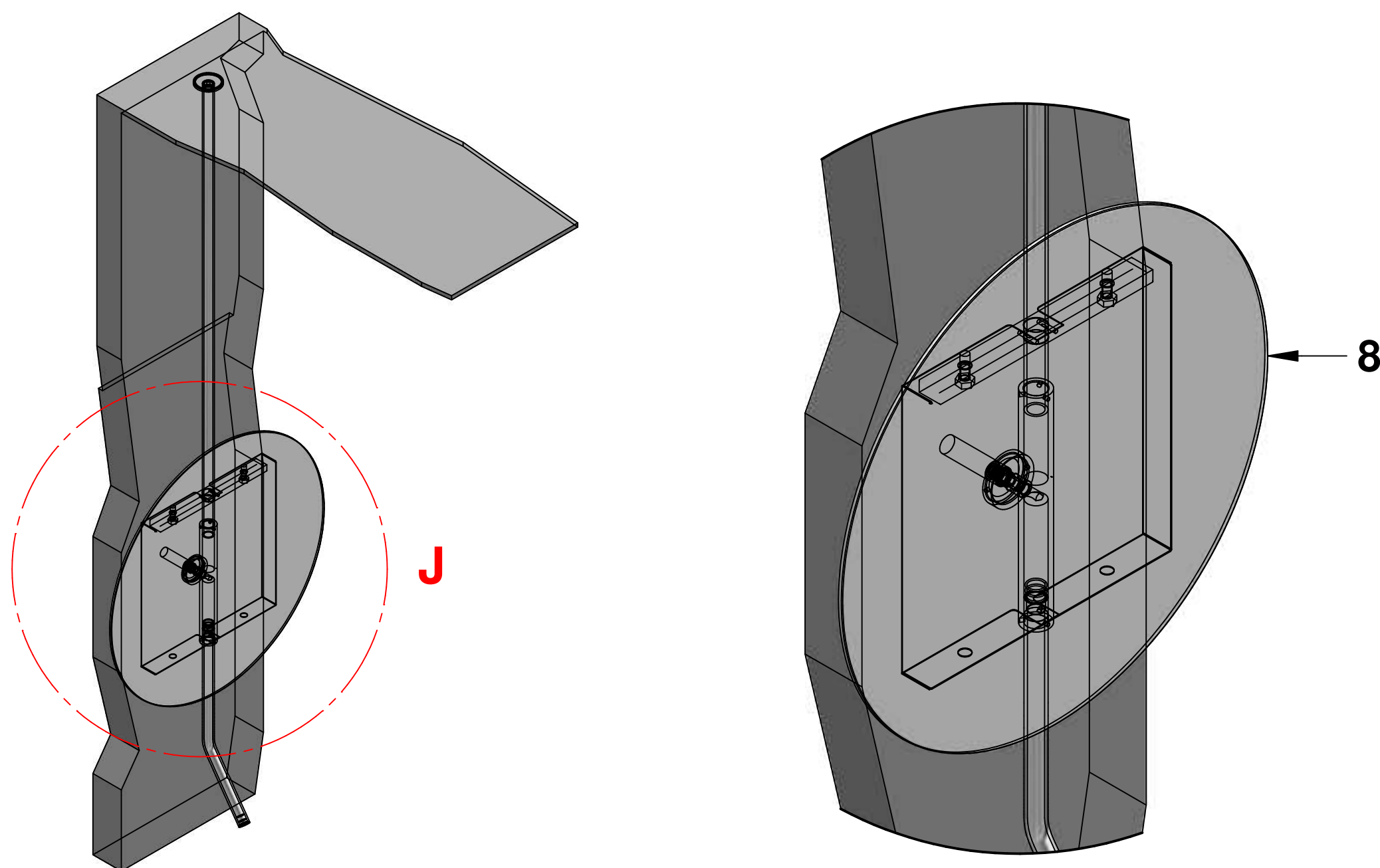
DETTAGLIO J
