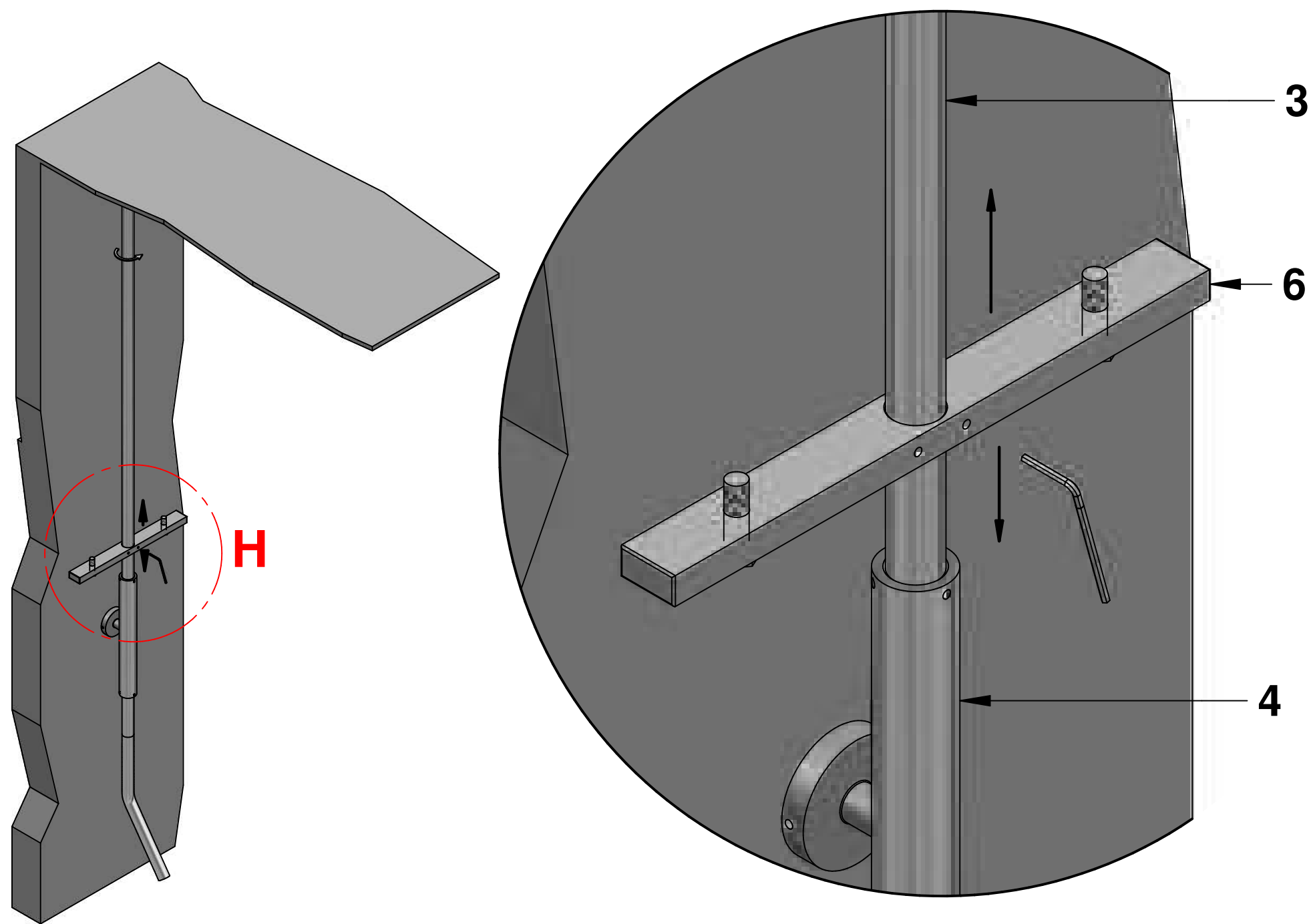
DETTAGLIO H
