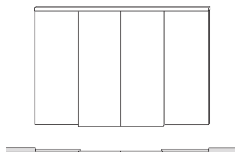
4 ante binario a 2 vie a soffitto 4 doors 2-way runners ceiling assembly 4 puertas vías con 2 vías de techo
