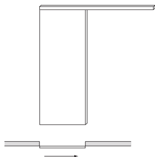
1 anta binario ad 1 via a parete 1 door 1-way runner wall assembly 1 puerta vía con 1 vía de pared
