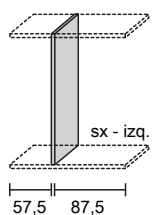
L. 147,5 dx o sx l/h or r/h - der.o izq.
