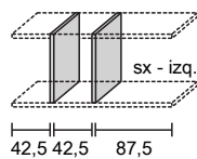
L. 177,5 dx o sx l/h or r/h - der.o izq.
