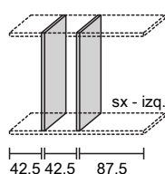
L. 177,5 dx o sx l/h or r/h - der.o izq.
