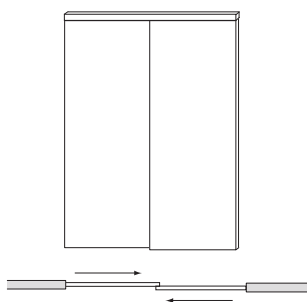
2 ante binario a 2 vie a soffitto 2 doors 2-way runners ceiling assembly 2 puertas vía con 2 vías de techo
