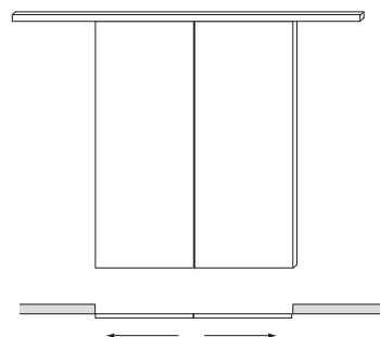
2 ante binario ad 1 via a parete 2 doors 1-way runner wall assembly 2 puertas vía con 1 vía de pared
