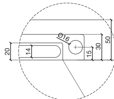
DETTAGLIO F
