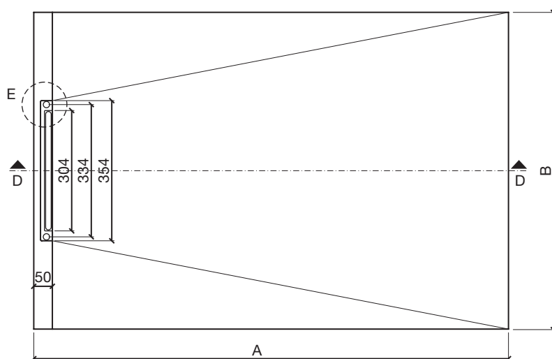
PIANTA
