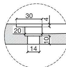
DETTAGLIO F
