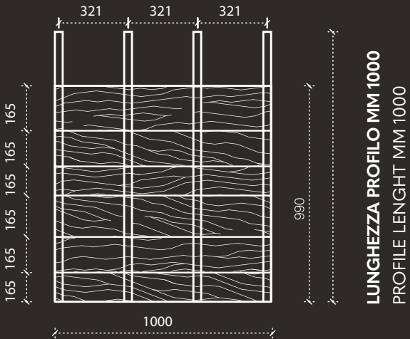
SCHEMA DI MONTAGGIO VERTICALE VERTICAL ASSEMBLY DIAGRAM EXAMPLE
