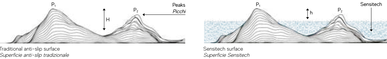
Surface section magnification (µm)* Ingrandimento di una sezione di superficie (µm)*
